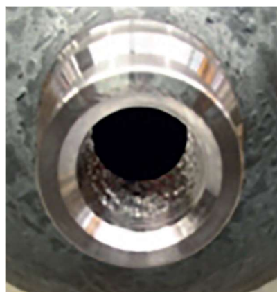
Рисунок А.13 – Выщербление резьбы
