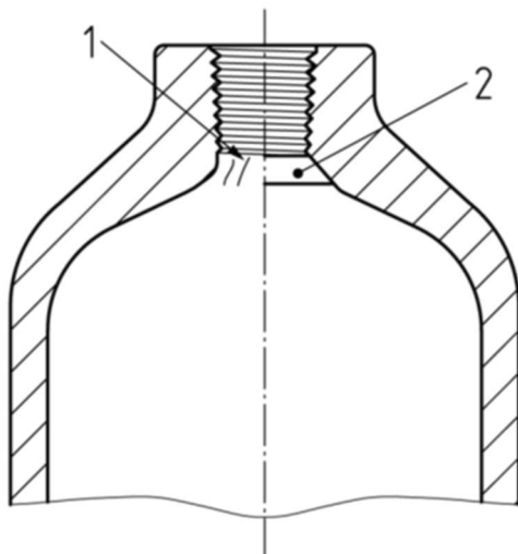
1 – складки или трещины; 2 – после механической обработки Рисунок А.9 – Складки или трещины на днище с горловиной до и после механической обработки
