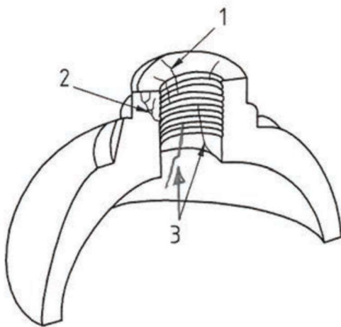
1 – трещины на торцевой поверхности горловины; 2 – поперечное сечение горловины с трещиной; 3 – распространение трещин на днище Рисунок А.7 – Трещины в горловине
