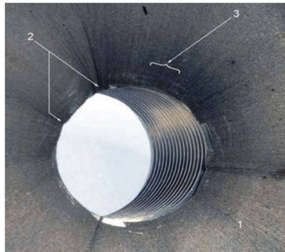
1 – область незначительных складок; 2 – средние складки; 3 – область круговых несовершенств Рисунок А.10 – Складки на днище
