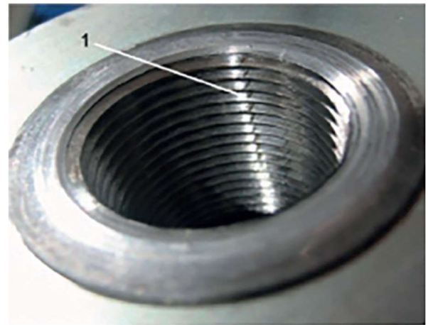
1 – неглубокая риска или царапина на резьбе горловины
