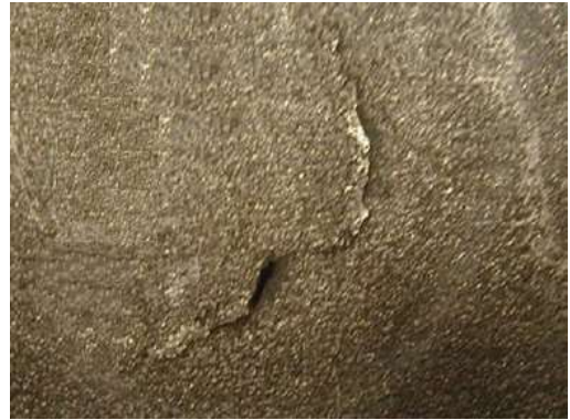
Рисунок А.6 – Характерный вид расслоения
