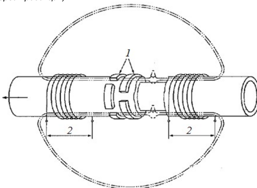
Рисунок 2 – Упрощенная схема определения поперечных дефектов методом рассеяния магнитного потока
