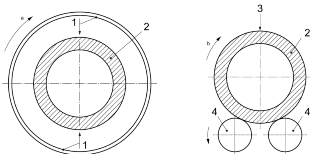
1 – положение преобразователя/дисковой катушки; 2 – труба; 3 – положение неподвижной дисковой катушки; 4 – ролики; a – направление вращения преобразователя; b – направление вращения трубы
