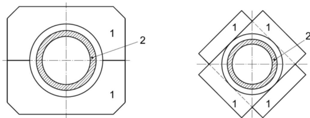
1 – сегментная катушка; 2 – труба
