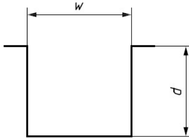
Рисунок 5 – Паз «N»-типа
