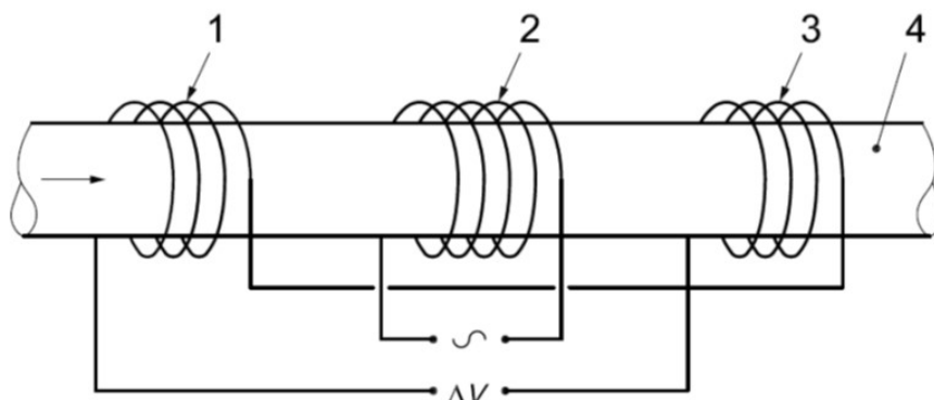
1 – вторичная катушка 1; 2 – первичная катушка; 3 – вторичная катушка 2; 4 – труба; ~ – переменный возбуждающий ток; \Delta V – выходной сигнал
