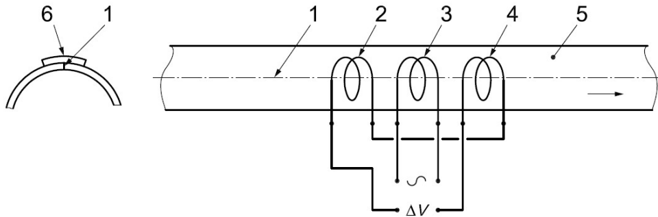
1 – сварной шов; 2 – вторичная катушка 1; 3 – первичная катушка; 4 – вторичная катушка 2; 5 – труба; 6 – катушка; ~ – переменный возбуждающий ток; \Delta V – выходной сигнал
