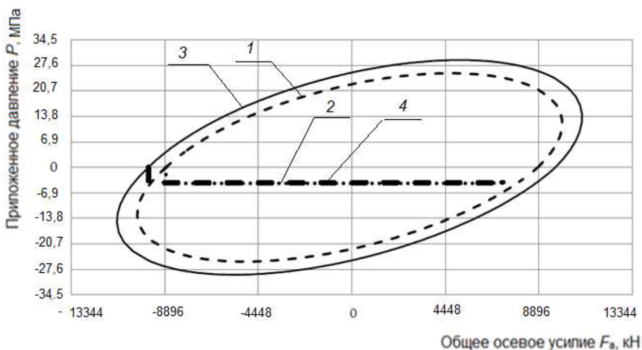
1 – кривая 1 a ; 2 – кривая 2 a ; 3 – кривая 4 a ; 4 – кривая 5 a
