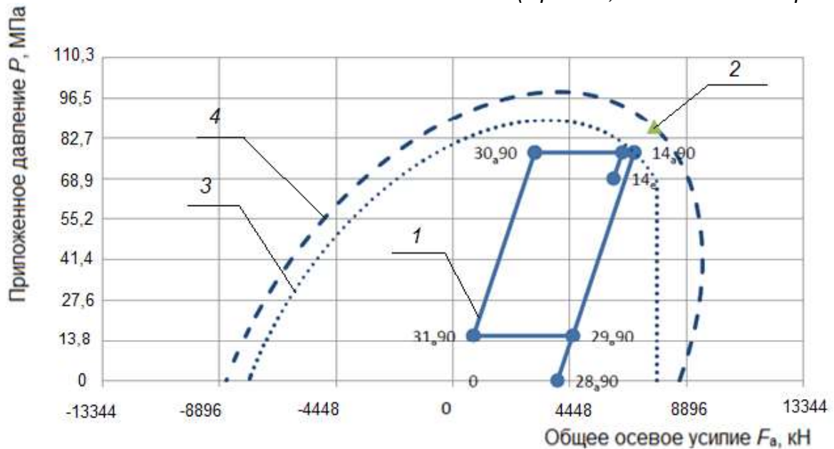
1 – точки TLE e ; 2 – точки CEE a ; 3 – 90% CEE a ; 4 – кривая 4 a
