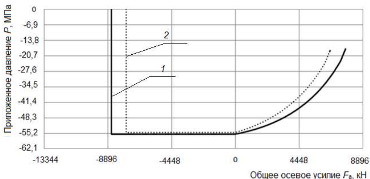
Рисунок D.8 – Кривые фактического (5 а ) и номинального (2 а ) давления смятия по API испытательного образца тела трубы при температуре окружающей среды
