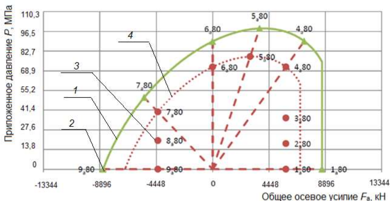
Рисунок D.16 – Точки CEE a и точки нагрузки 80 % TLE a при температуре окружающей среды
