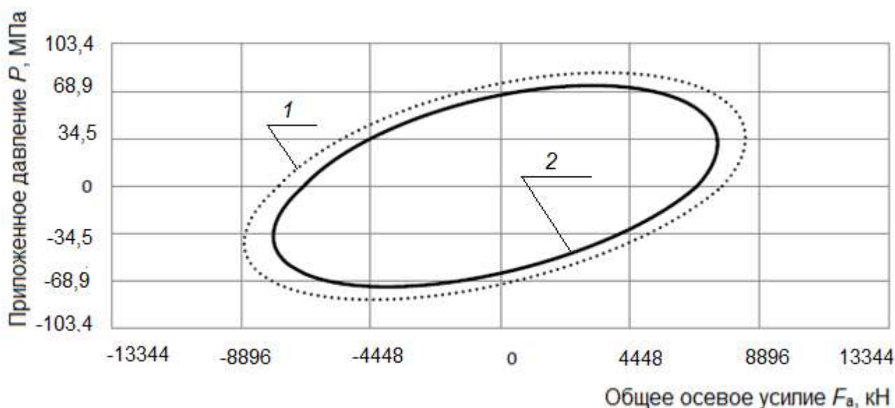
1 – кривая 1 а ; 2 – кривая 1 е
