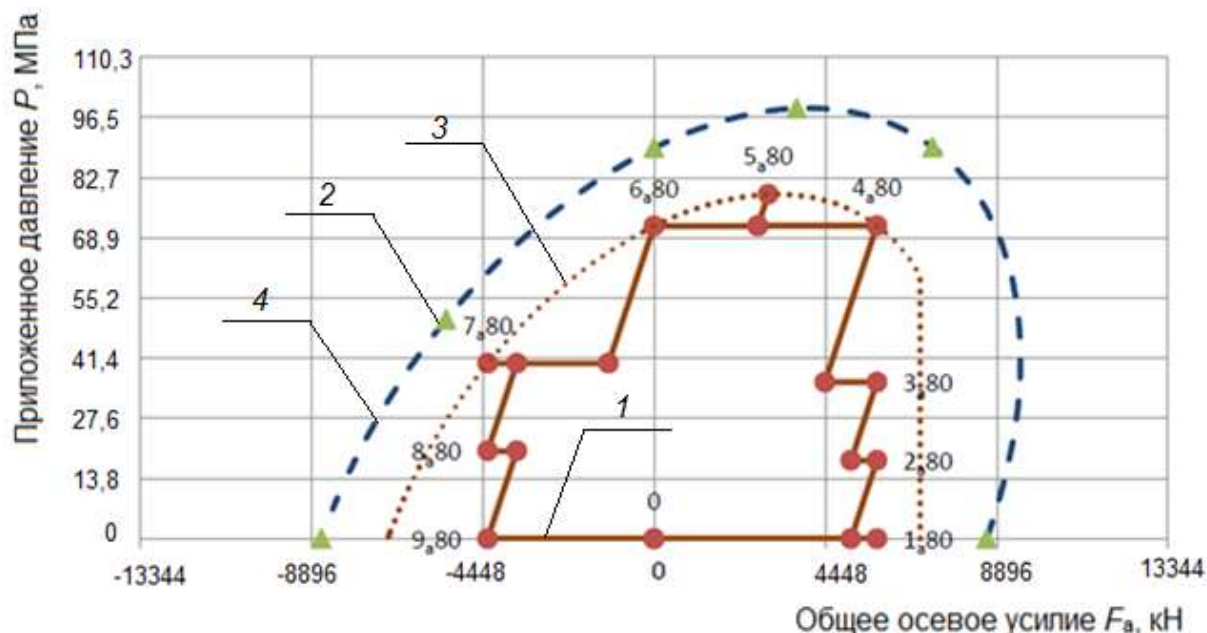
Рисунок D.20 – B a 80 % (QI, QII), TS-B этапы нагрузки 1 – 19
