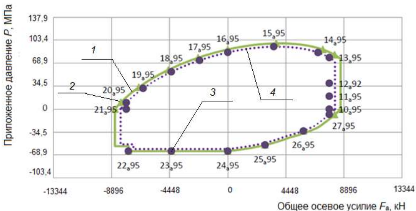
Рисунок D.17 – Точки CEE a и точки нагрузки 95 % TLE a при температуре окружающей среды
