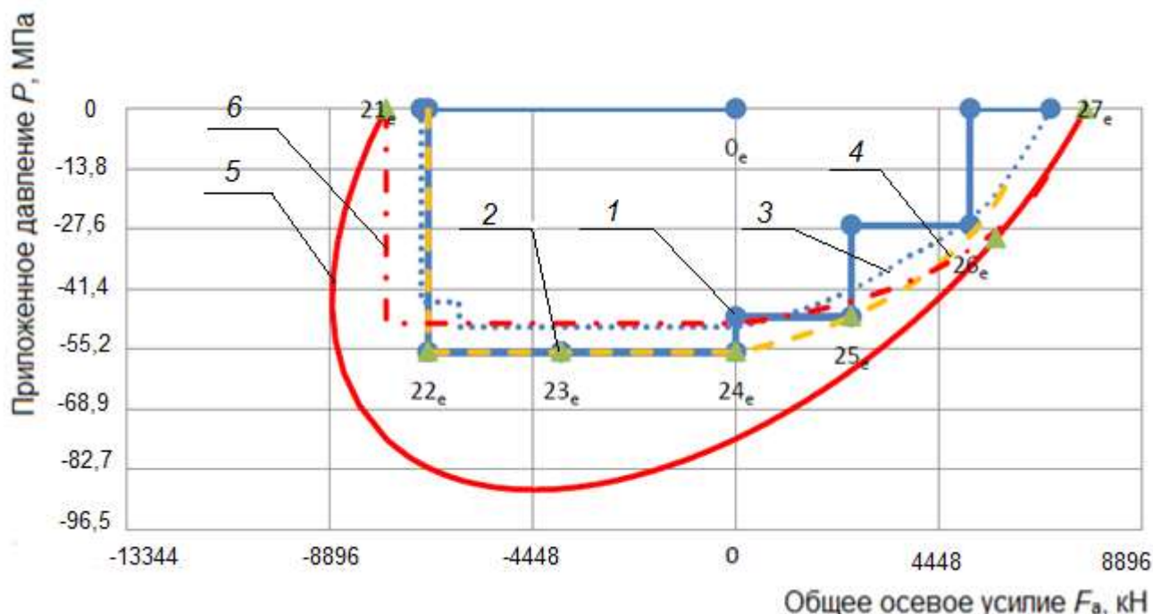
Рисунок D.27 – A e 90 % (QIII, QIV) и A e 90 % (QIV, QIII), TS-A этапы нагрузки 25 – 51
