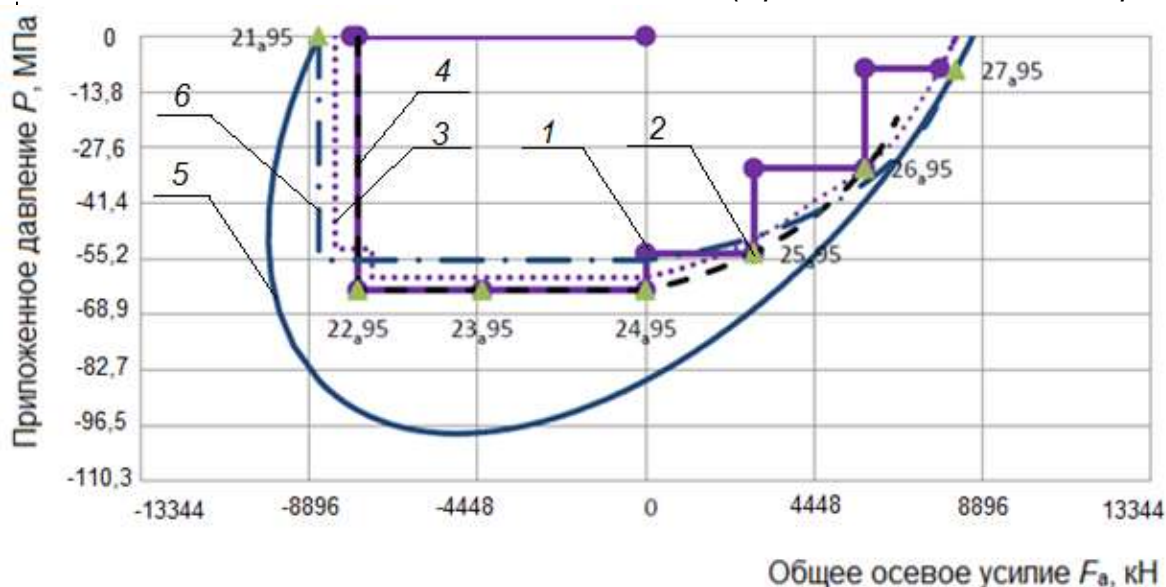
Рисунок D.34 – A a 95 % (QIII, QIV) и A a 95 % (QIV, QIII), TS-A этапы нагрузки 222 – 248
