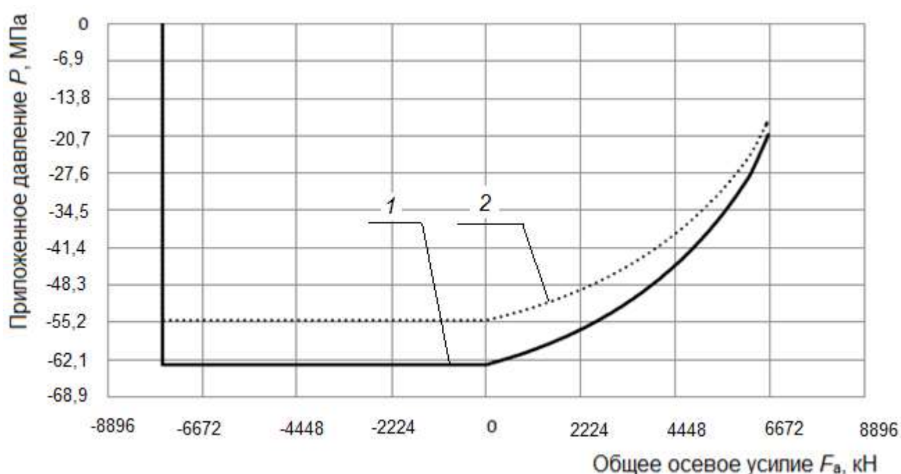
1 – кривая 3 а ; 2 – кривая 2 а
