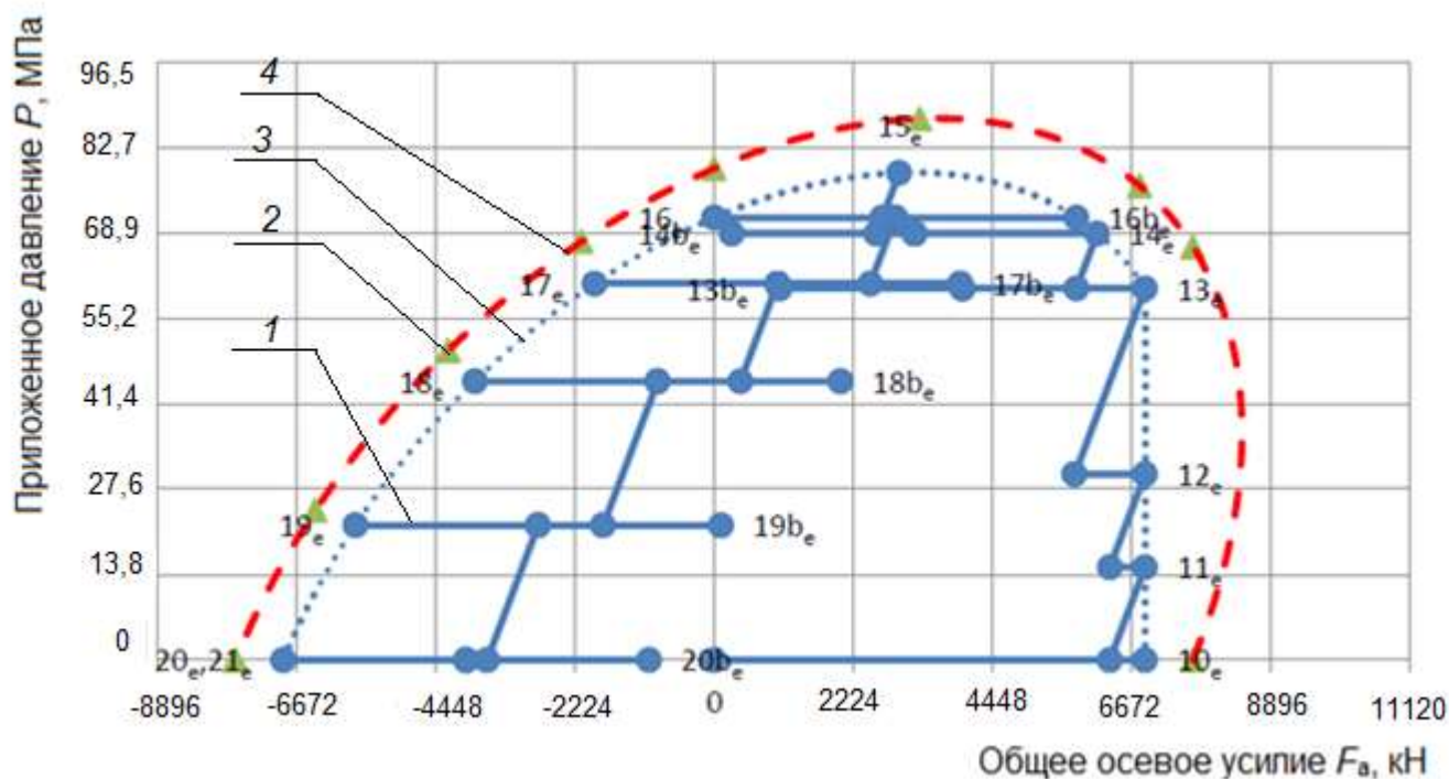
Рисунок D.22 – V_b 90 % (QI, QII, QI), TS-B этапы нагрузки 67 – 155
