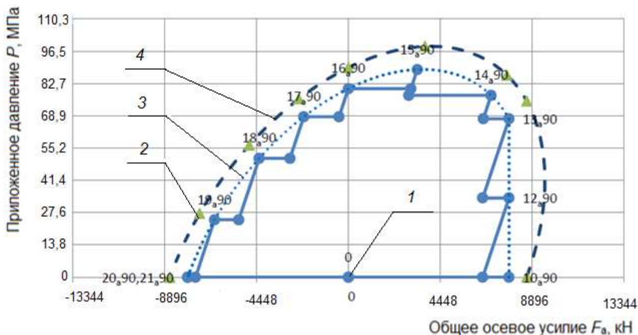
1 – точки TLE a 90; 2 – точки CEE a ; 3 – 90% CEE a ; 4 – кривая 4 a
