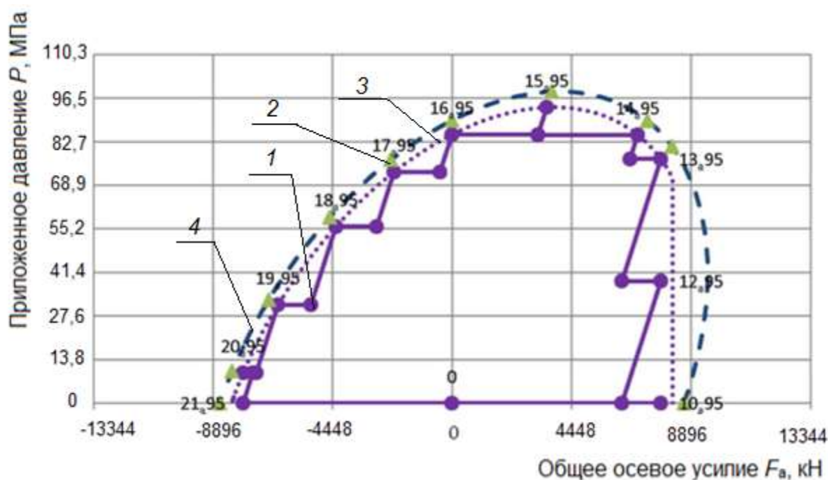
1 – точки TLE a 95; 2 – точки CEE a ; 3 – 95 % CEE a ; 4 – кривая 4 a
