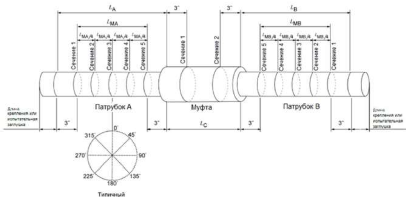
Рисунок D.3 – Места измерений
