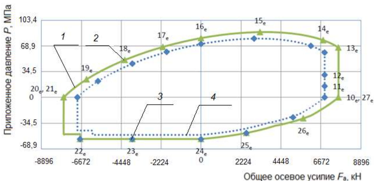
Рисунок D.19 – Точки 90 % CEE e и точки нагрузки TLE e при повышенной температуре
