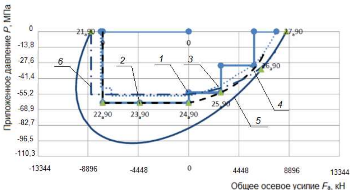
1 – точки TLE a 90; 2 – точки CEE a ; 3 – 90 % CEE a ; 4 – кривая 3 a ; 5 – кривая 4 a ; 6– кривая 5 a
