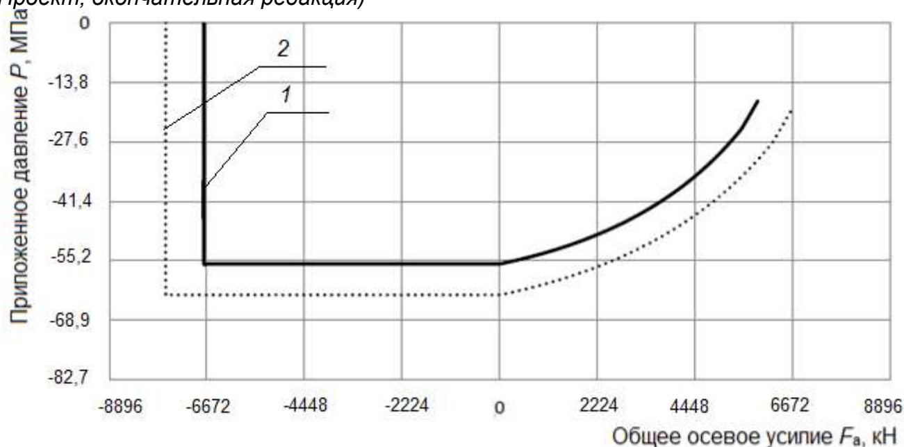
1 – кривая 3 е ; 2 – кривая 3 а
