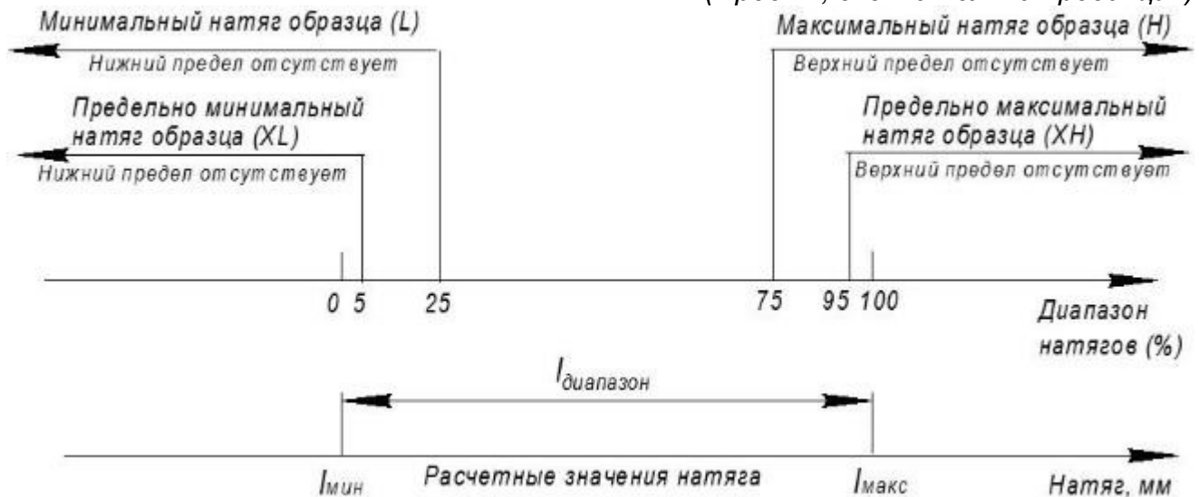
Рисунок 19 – Схематическое изображение диапазона натягов испытательных образцов
