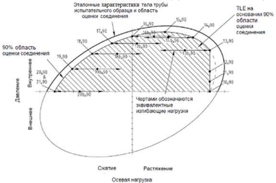
Рисунок 31 – Пример точек нагрузки TS-B при температуре окружающей среды с изгибом при величине нагрузки 90 % от СЕЕ, при совпадении эталонных характеристик тела трубы и области оценки резьбового соединения
