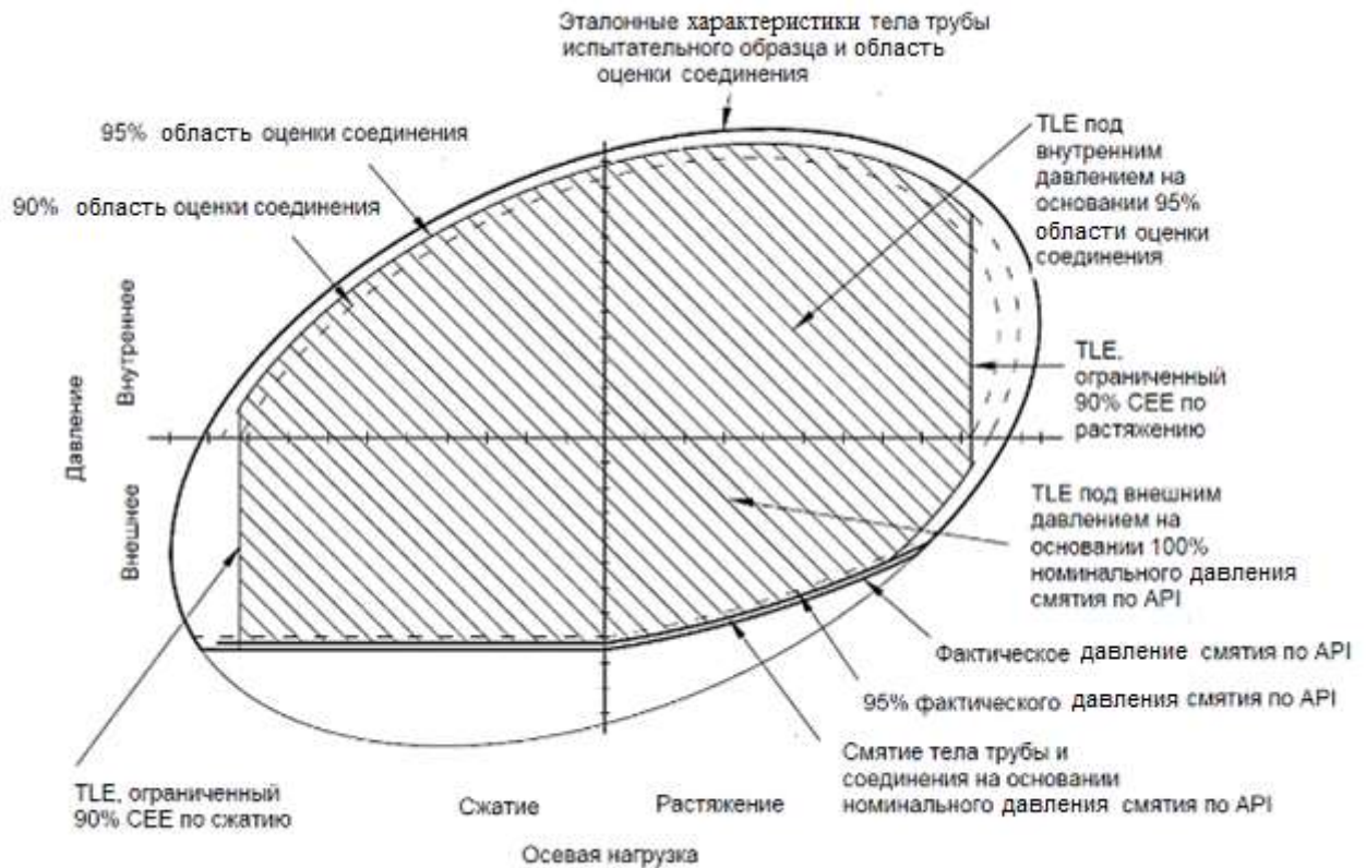
Рисунок 21 – Пример области испытательных нагрузок при совпадении эталонных характеристик тела трубы и области оценки резьбового соединения, и при TLE, составляющей 95 % от CEE для внутреннего давления и 100 % от номинального давления смятия по API для наружного давления
