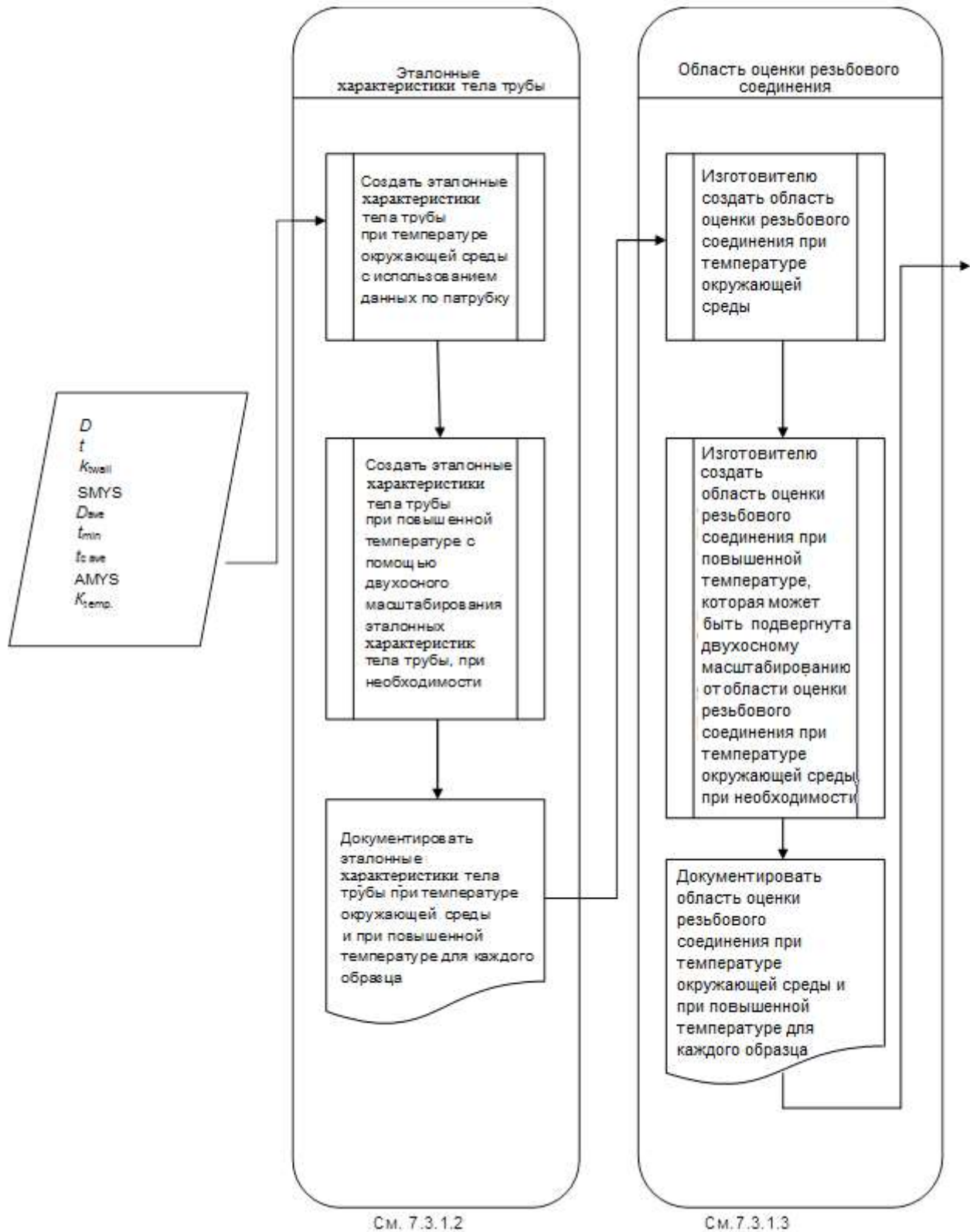
Рисунок 2 – Схема определения эталонных характеристик тела трубы при температуре окружающей среды и при повышенной температуре, и области оценки резьбового соединения для испытательного образца
