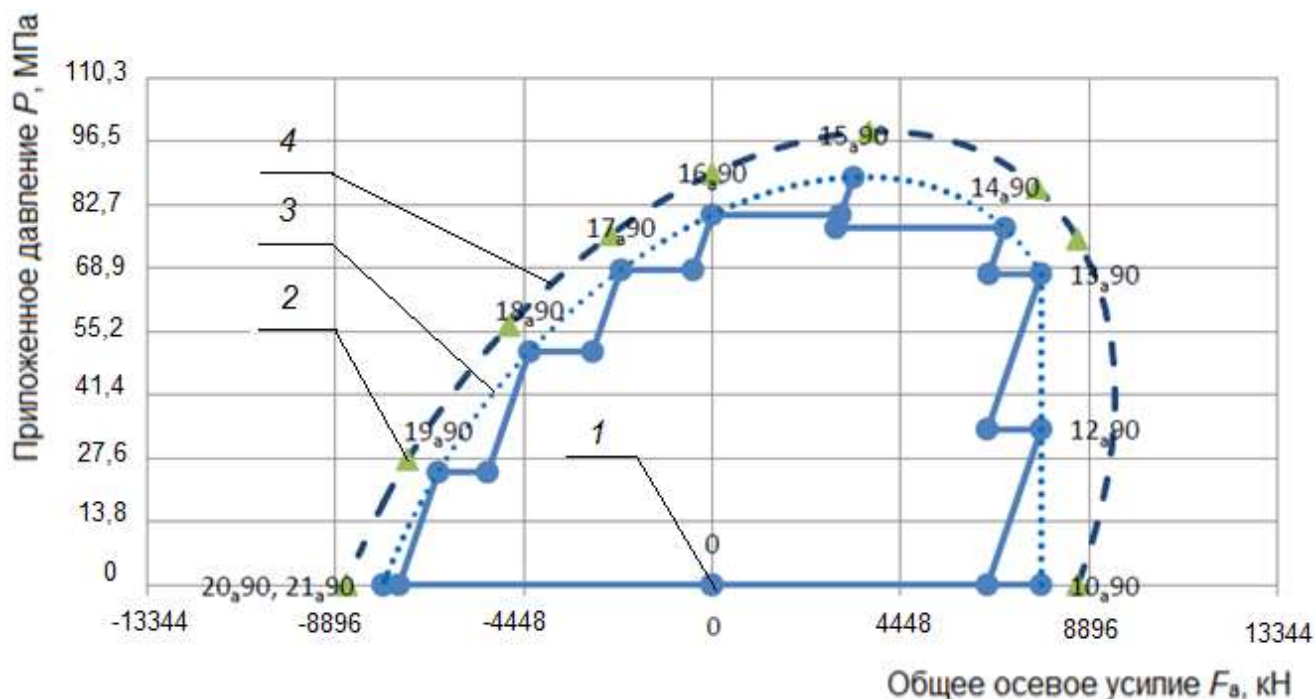
Рисунок D.32 – A a 90 % (QI, QII), TS-A этапы нагрузки 176 – 198
