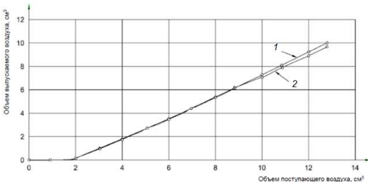
Рисунок 12 – Пример графика оценки чувствительности системы выявления утечек
