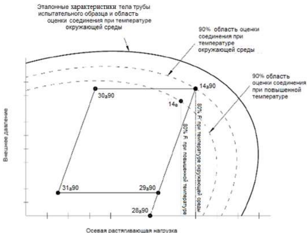
Рисунок 34 – Процедура расчета траектории нагрузки при проведении TS-C
