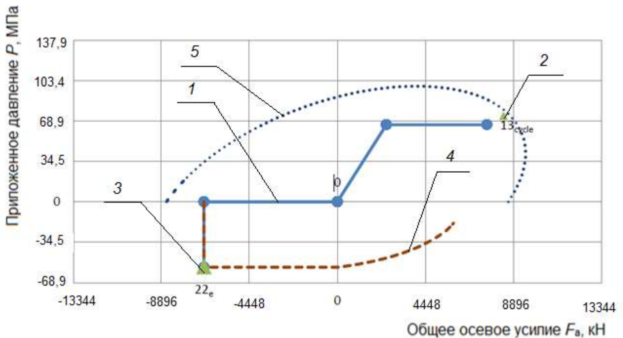
Рисунок D.29 – A e 90 % пять циклов QI – QIII, TS-A этапы нагрузки 75 – 125
