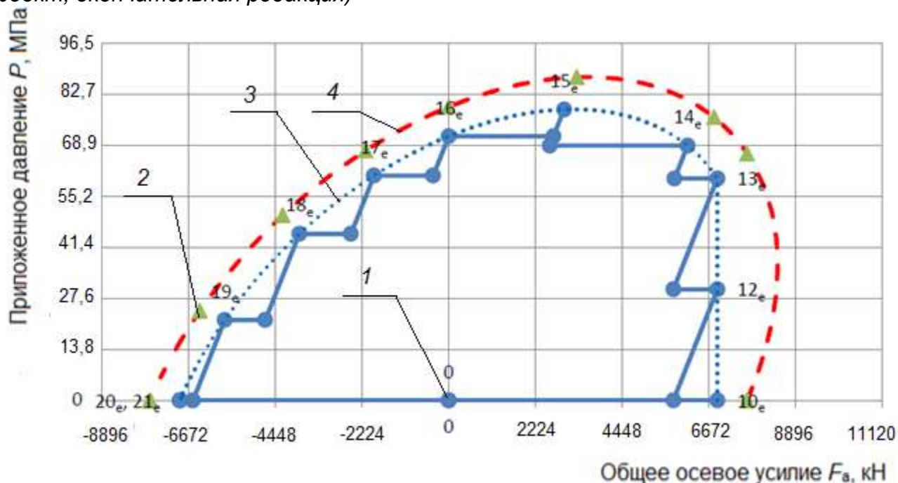
Рисунок D.28 – A e 90 % (QIII, QIV) и A e 90 % (QIV, QIII), TS-A этапы нагрузки 52 – 74
