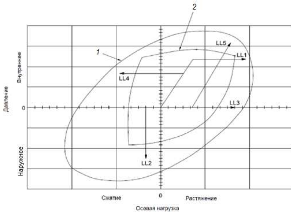
1 – 100 % VME области предела текучести тела трубы; 2 – 100 % области оценки резьбового соединения Рисунок 36 – Траектории приложения нагрузки при испытании при предельных нагрузках (пример 2)
