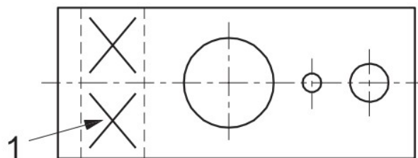
б – IQI ступенчатый с отверстиями
