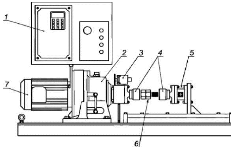
Рисунок 1.3 — Установка для испытания резьбовой смазки
