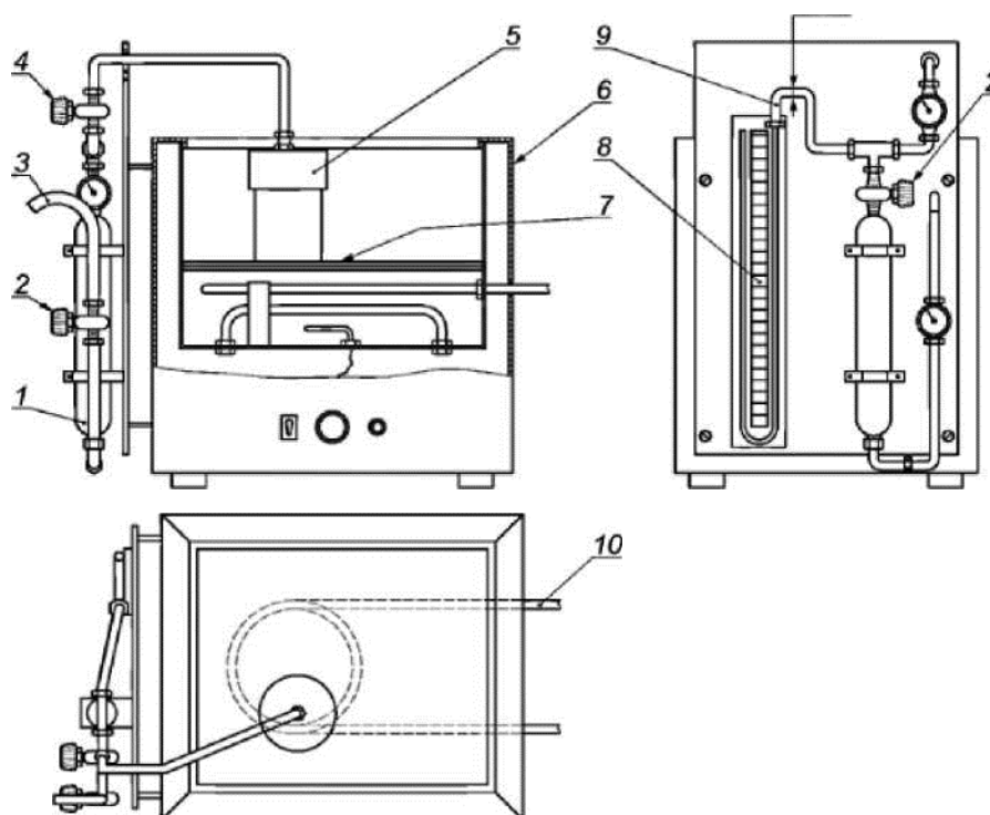
Рисунок G.1 — Пример 1 установки для измерения выделения газа
