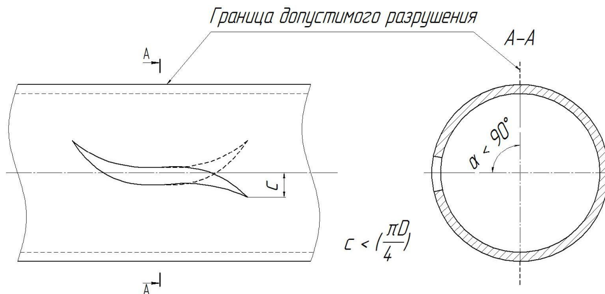
Рисунок 11 – Допустимый профиль разрыва – продольный разрыв с одним ответвлением
