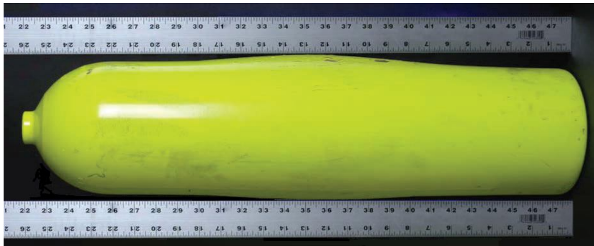
Рисунок А.2 – Вздутие баллона
