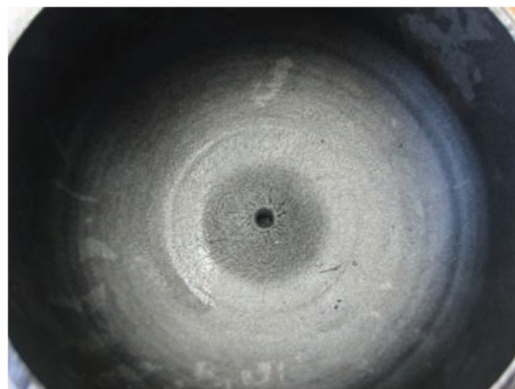
Рисунок А.13 – Возможный дефект в глухом днище баллона, изготовленного из трубной заготовки
