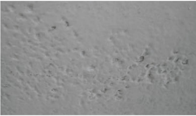
Рисунок А.18 – Питтинговая коррозия
