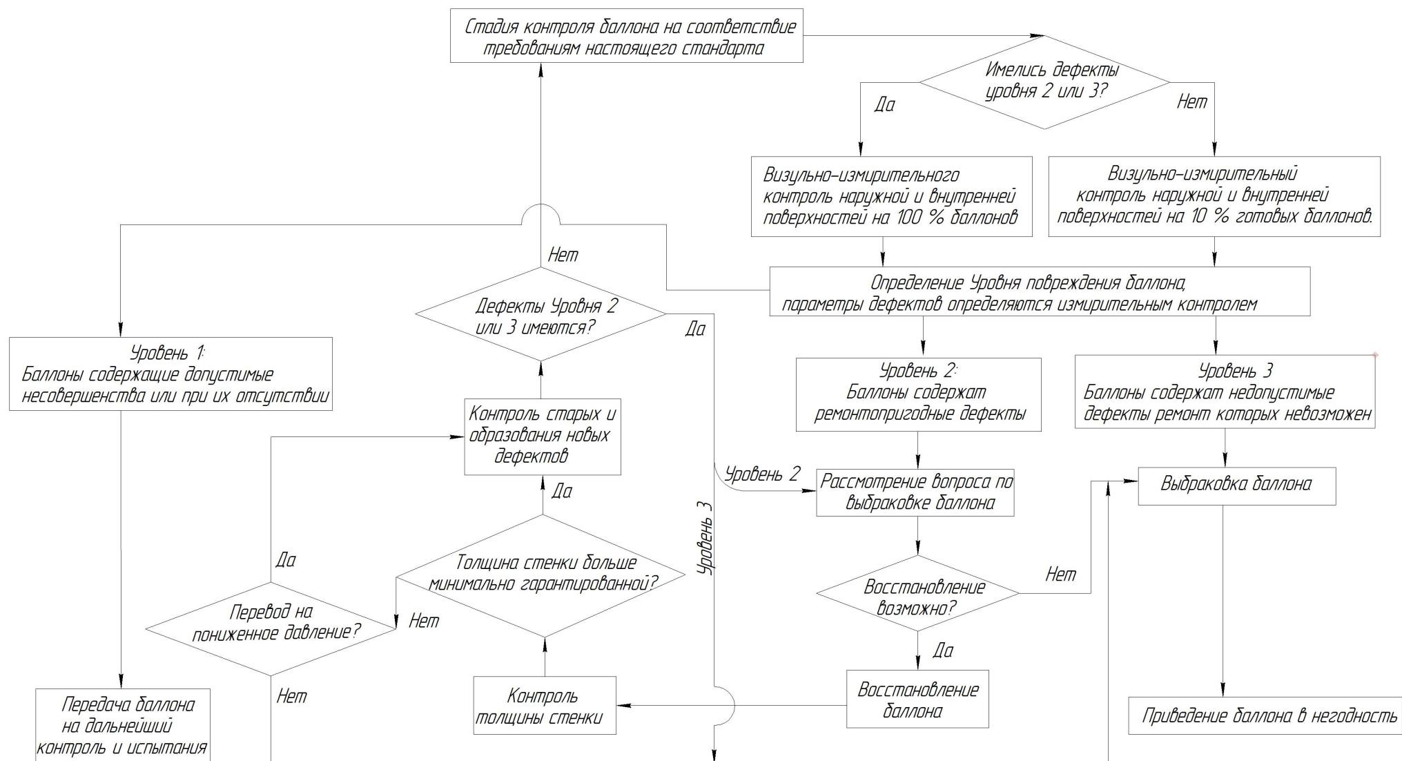
Рисунок А.1 – Схема проведения визуального и измерительного контроля наружной и внутренней поверхностей баллонов
