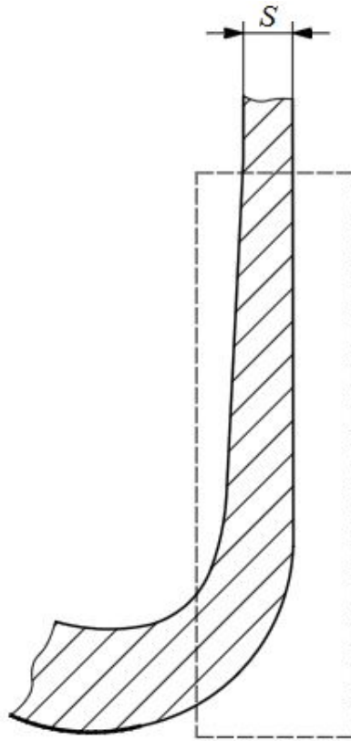
Рисунок Б.1 – Переходная зона между днищами и цилиндрической частью баллона
