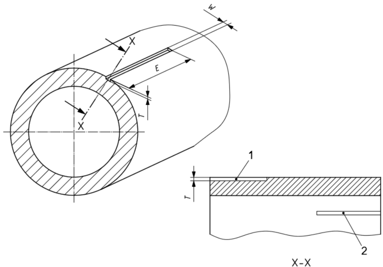
Рисунок Б.3 – Форма и размеры искусственных отражателей, применяемых для обнаружения продольных несовершенств
