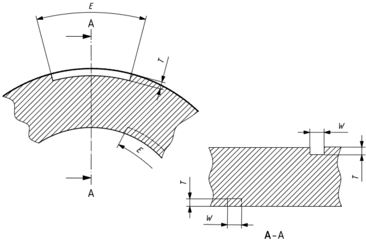
Рисунок Б.4 – Схема искусственных отражателей, расположенных по окружности
