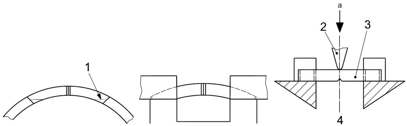
Рисунок 7 – Ориентация поперечных и продольных образцов для испытания на ударный изгиб
