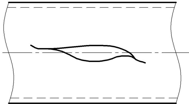
Рисунок 10 – Допустимый профиль разрыва – продольный разрыв без ветвления
