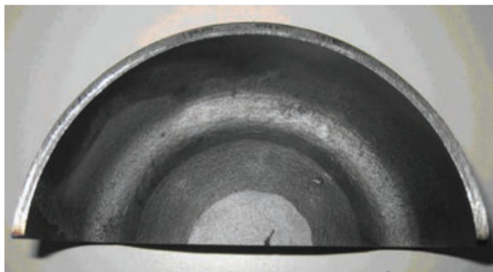
Рисунок А.13 – Возможный дефект в глухом днище баллона, изготовленного из трубной заготовки
