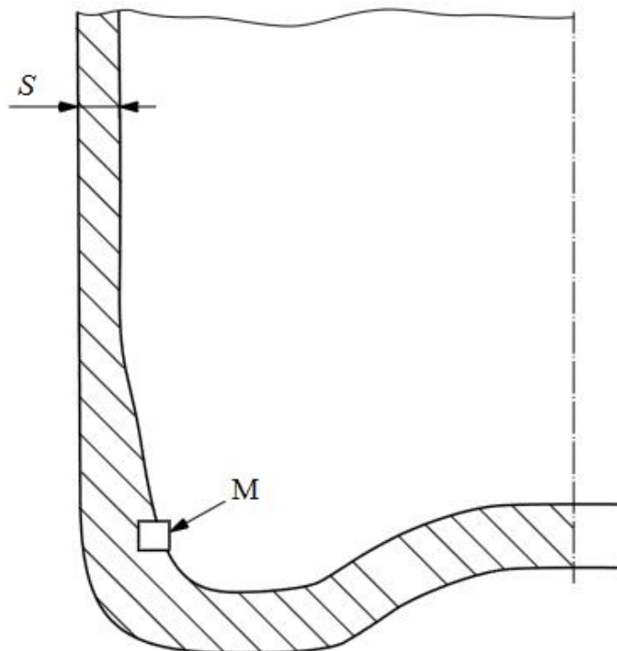
Рисунок Б.2 – Схематичное представление искусственные отражатели для стандартных образцов
