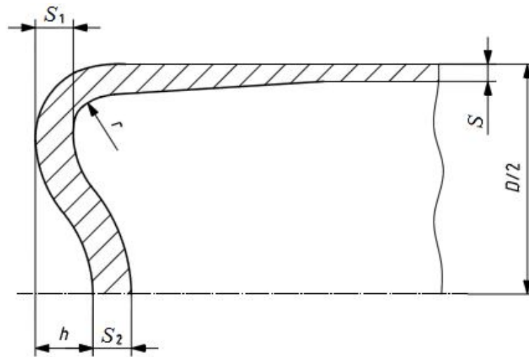
Рисунок 2 – Вогнутое днище баллона
