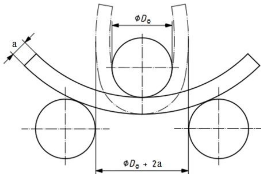
Рисунок 6 – Испытание на изгиб
